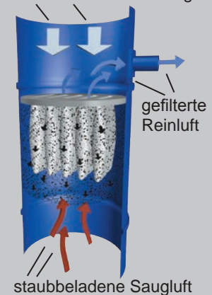
AirShock®-Filterabreinigung
